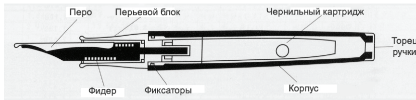
Рис. 1.: а — перьевая ручка (общий вид); б — увеличенное изображение пишущего узла перьевой ручки; в — строение перьевой ручки
